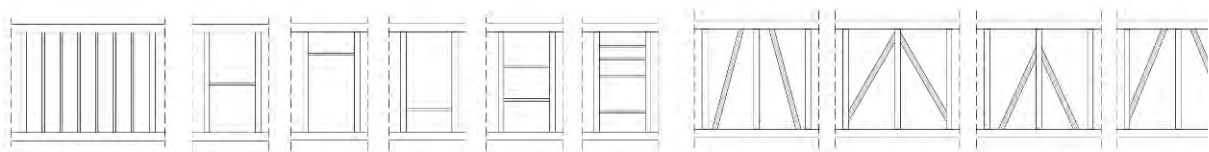
Figura 5. Esquemas simplificados de los diferentes tipos de elementos estructurales intermedios verticales, horizontales y diagonales.
