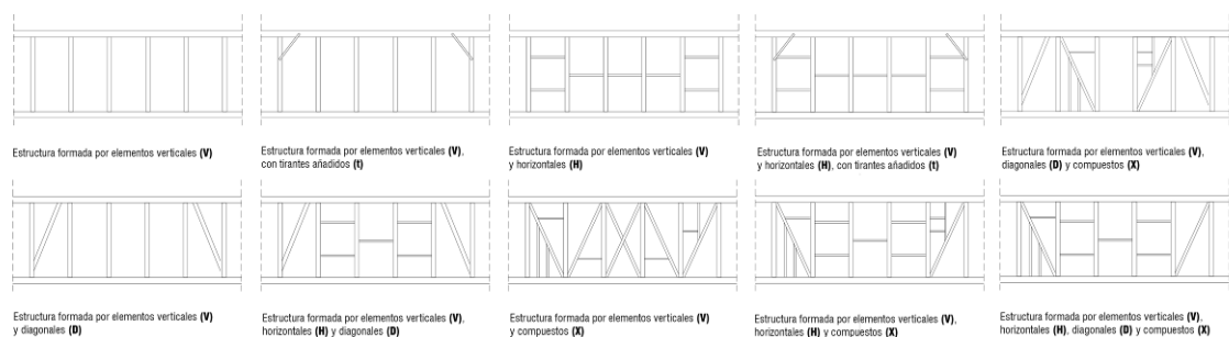
Figura 3. Esquemas simplificados de los diferentes tipos de geometría estructural.
