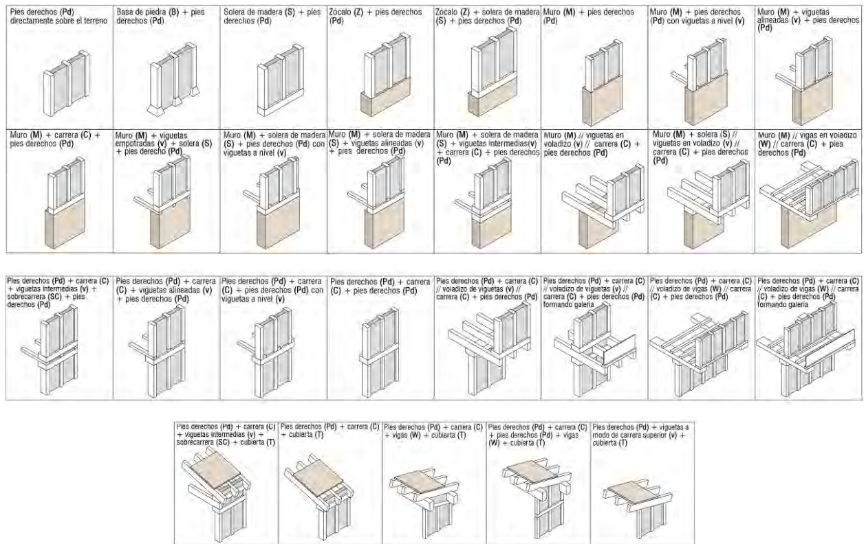
Figura 4. Esquemas simplificados de los diferentes tipos de encuentros del elemento entramado con otros elementos constructivos: extremo inferior, encuentros interiores y extremo superior.
